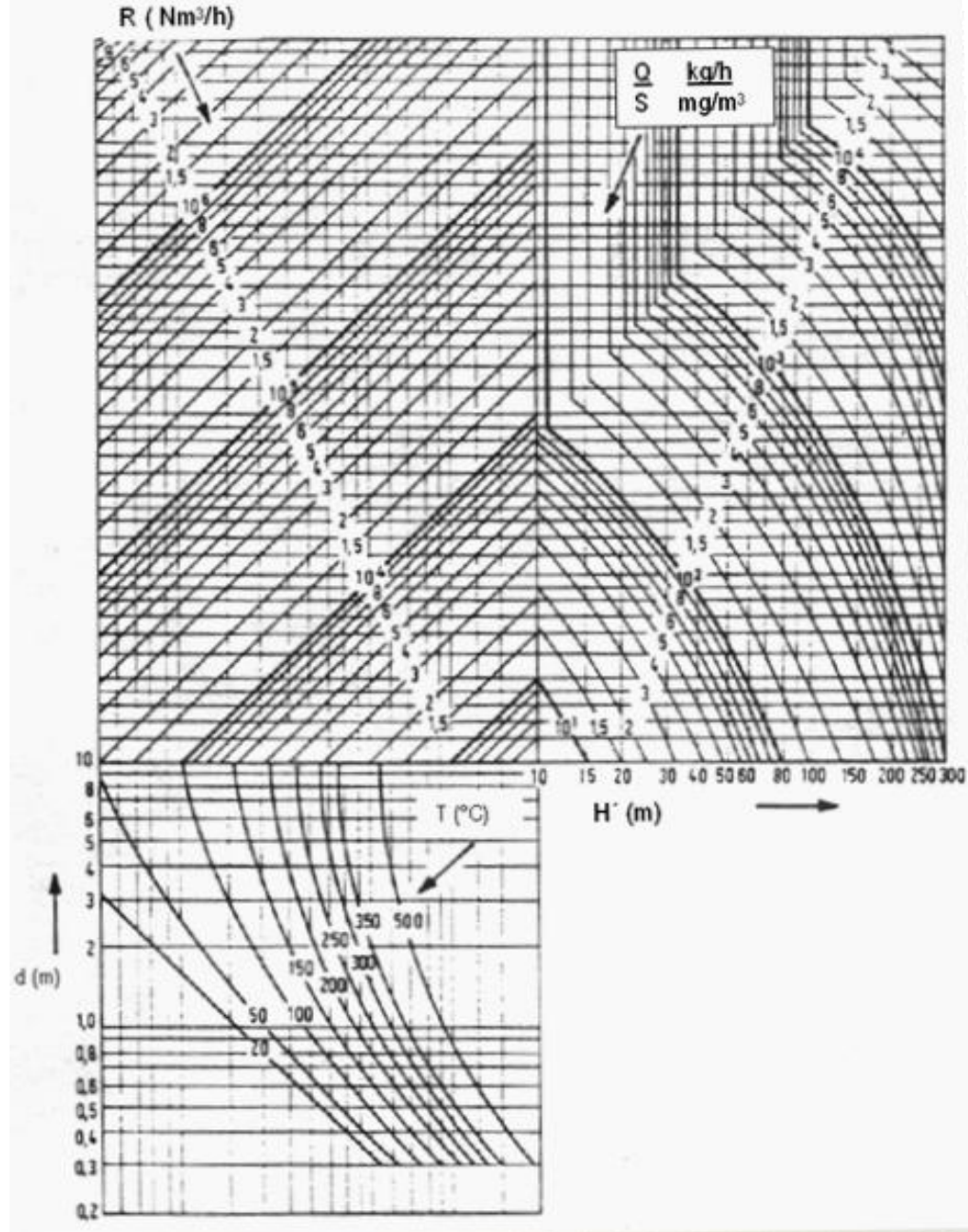
Gráfica 1. Nomograma para el cálculo de la altura mínima de chimenea.
